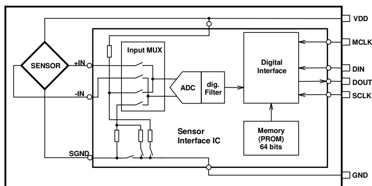
图1: MS5534C电路图
